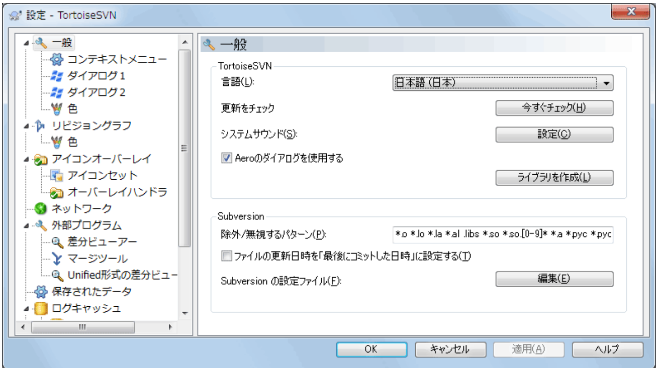
図4.68 設定ダイアログの「全般」ページ
