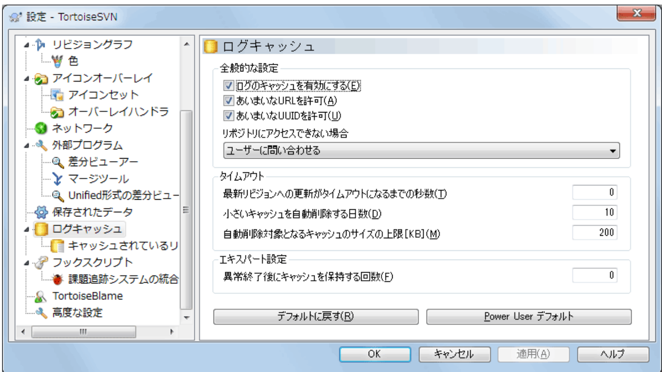
図4.83 設定ダイアログの「ログキャッシュ」ページ
