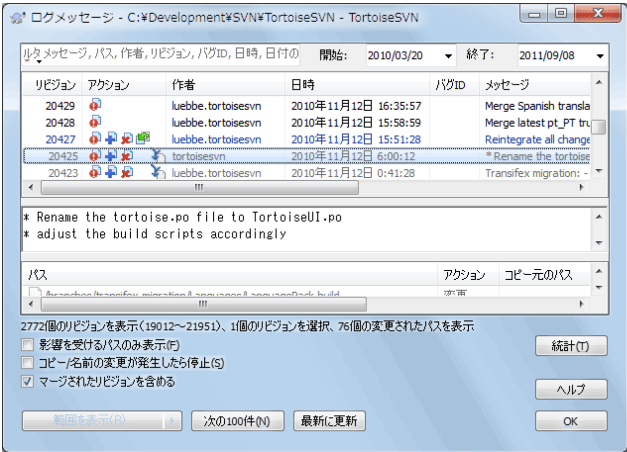
図4.22 マージ追跡リビジョンを表示したログダイアログ
