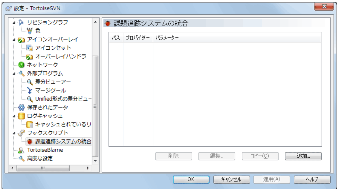
図4.87 設定ダイアログの「課題追跡システムとの統合」ページ
