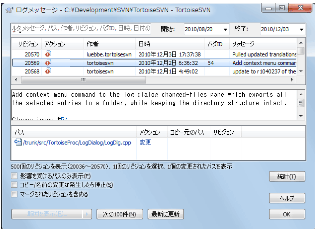
図4.16 リビジョンログダイアログ
